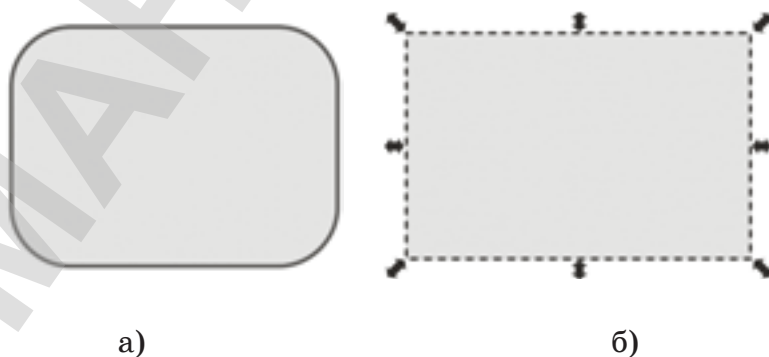
Рис. 31. Редактирование кривых
