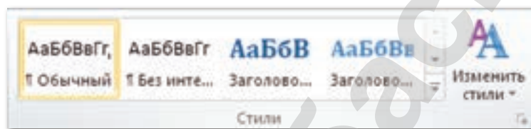
Рис 55. Стили заголовков
