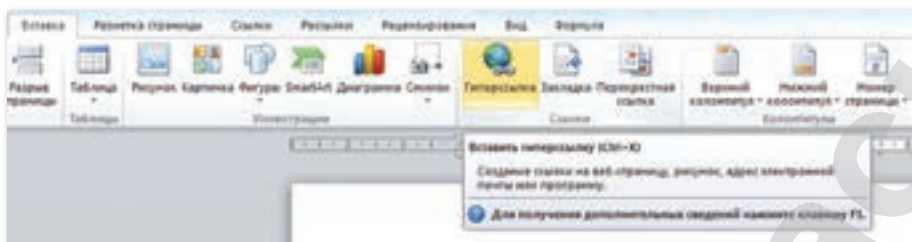
Рис. 52. Вставить гиперссылку
