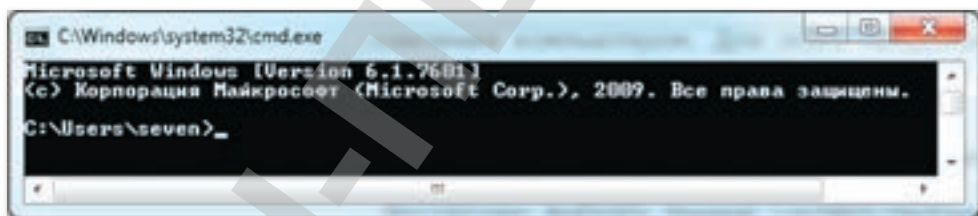
Рис. 12. Командный интерфейс
