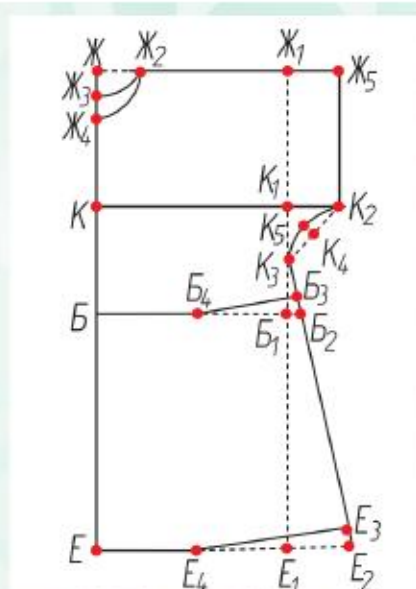
Жеңі тұтас пішілген иықты бұйымның сызбасы
