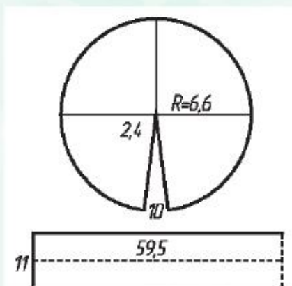
Тақияның сызбасы
