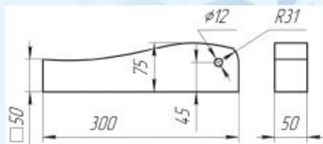
Үстел аяғының сызбасы
