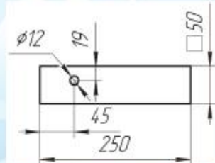
Бекітпенің сызбасы
