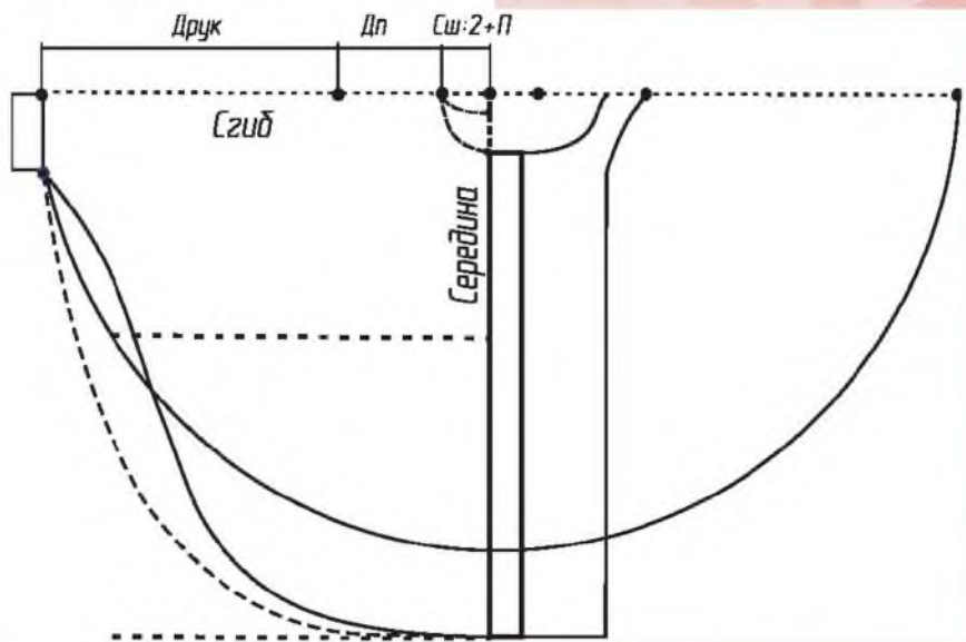
Моделирование пончо, туники
