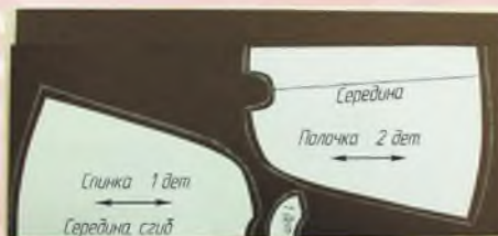
Раскладка выкроек с цельнокроеным подбортом
