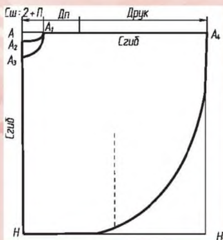
Чертеж пончо, туники
