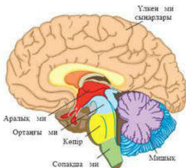
182-сурет. Мидың ұзынынан кесіліп көрсетілген негізгі бөлімдері
