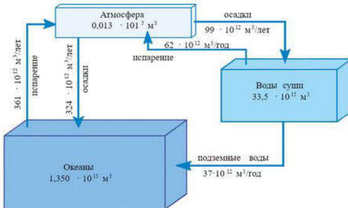
Рис. 4. Цифровая модель мирового водного баланса
