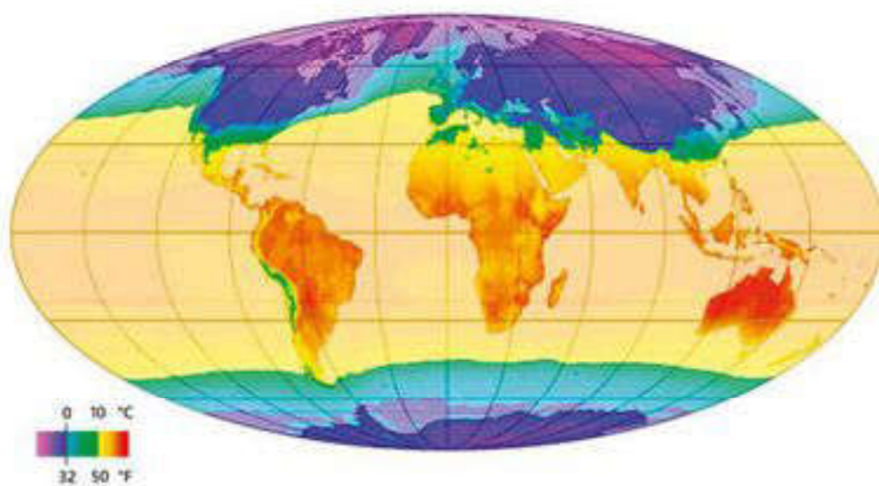
Рис. 12. Радиационный баланс января
