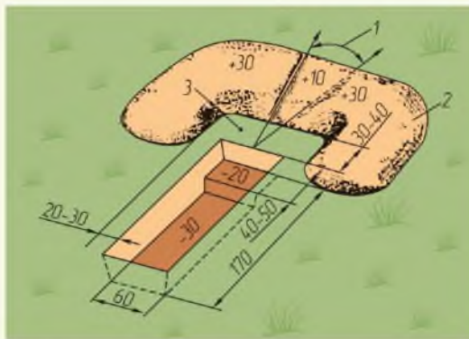
Рисунок 1.13. Одиночный окоп для стрельбы из автомата лежа: 1 – сектор обстрела; 2 – бруствер; 3 – берма
