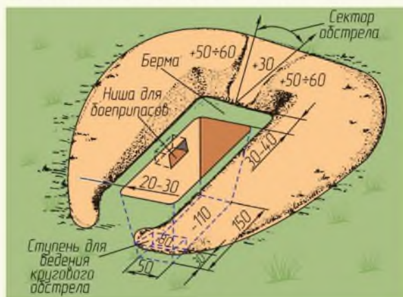
Рисунок 1.14. Окоп для стрельбы из автомата стоя
