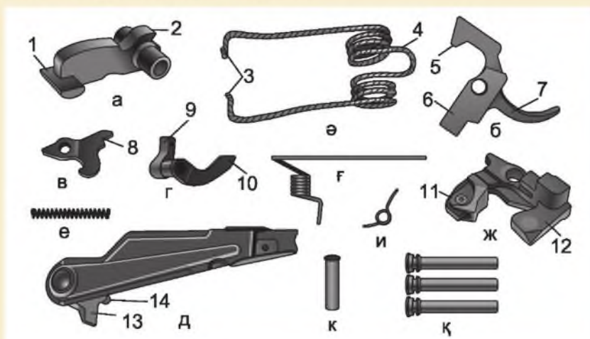
4.21-сурет. Соққыш-ағытқыш механизмнің бөлшектері: а – шүріппе; ә – атқарушы серіппе; б – ағытқыш ілмек; в – дара атуға арналған автоағытқыш тежеуіші; г – автоағытқыш; ғ – автоағытқыш серіппесі; д – ауыстырғыш; е – дара ату тежеуішінің серіппесі; ж – шүріппе баяулатқыш; и – шүріппе баяулатқышының серіппесі; к – түтікше ось; қ – осьтер; 1 – соққылық ендіргіш; 2 – автоағытқыш ендіргіші; 3 – бүгілген ұшы; 4 – ілмек; 5 – пішінді дөңес; 6 – тікбұрышты дөңес; 7 – ағытқыш құйрықша; 8 – ойық; 9 – тежеуіш (шептало); 10 – иінтірек; 11 – ілгіш; 12 – алдыңғы дөңес; 13 – сектор; 14 – шетмойын
