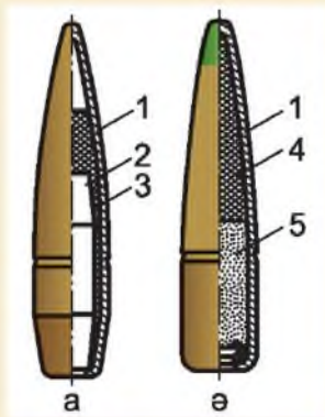
4.27-сурет. Оқтар: а – болат өзекті қарапайым оқ; б – жарқырағыш оқ;
