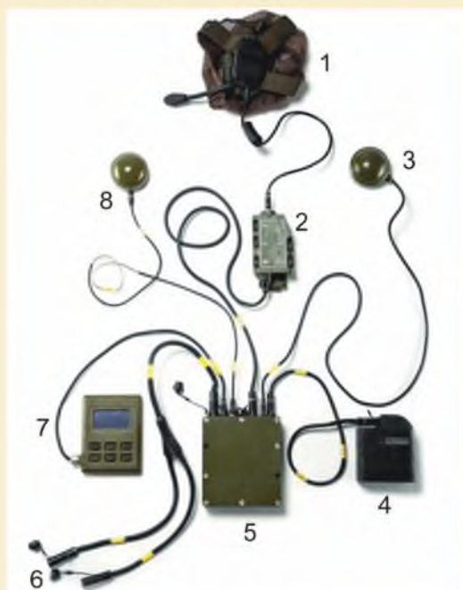
6.8-сурет. Жергілікті жерде бағдар алу жабдықтарының кешені: 1 – белсенді шу басушы гарнитура (құлаққап); 2 – жедел басқару пульті; 3 – жерсеріктік навигациялық жүйе; 4 – электр қоректендіруші контейнер (аккумулятор батареясы); 5 – аппараттық контейнер; 6 – қашықтық өлше- гіш, бұрыш өлшегіш сияқты аспаптарды қосатын шоғырсымдар; 7 – көпфункционалы пульті; 8 – жеке радиобайланыс модулі
