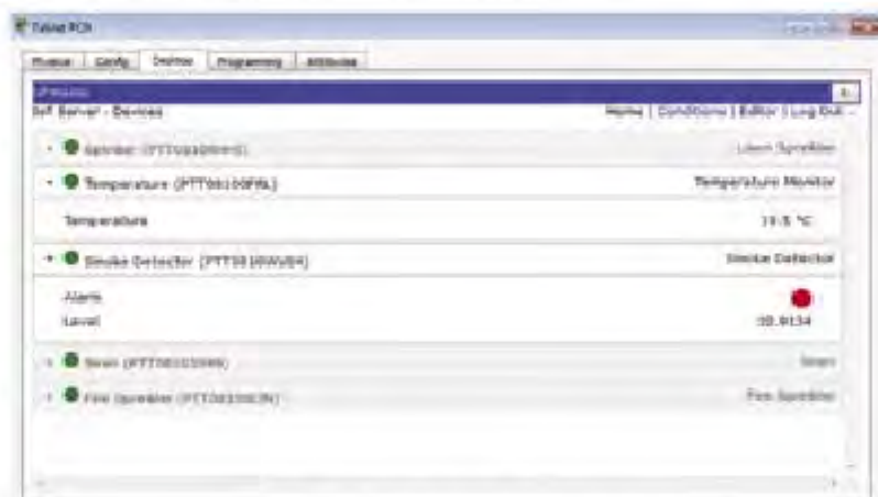
Рис. 4.3.22. IoT Monitor
