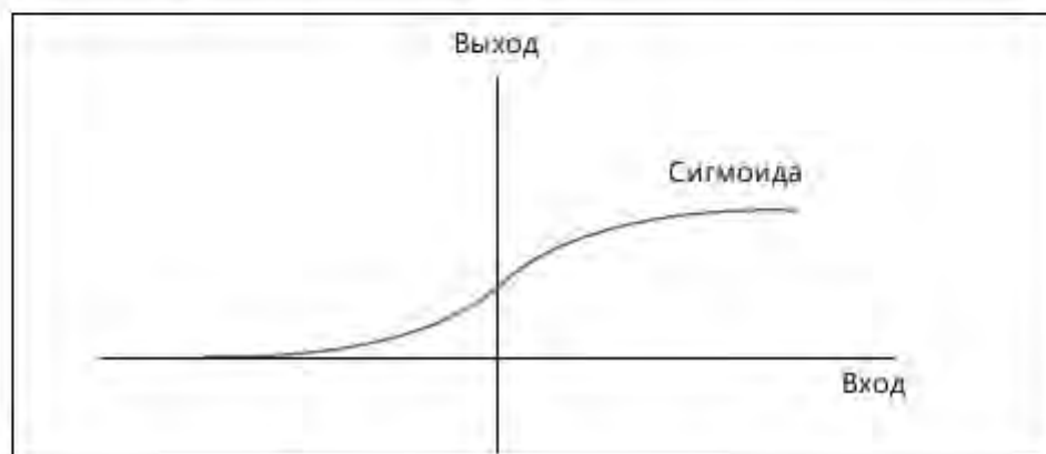
Рис. 1.4.1. S-образная сигмоида
