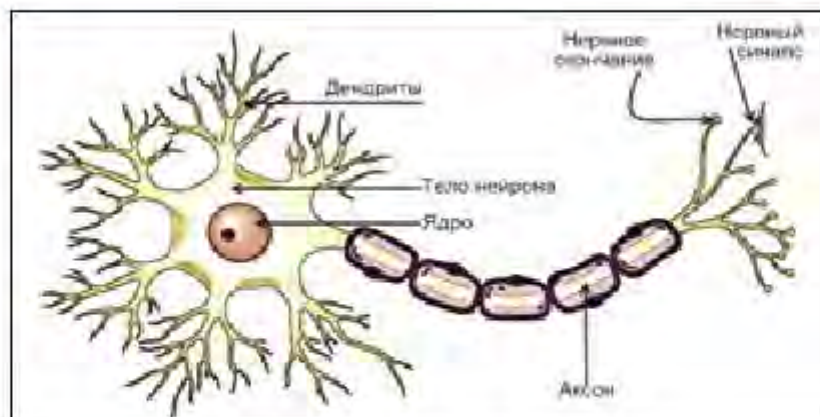
Рис. 1.3.1. Строение нейрона
