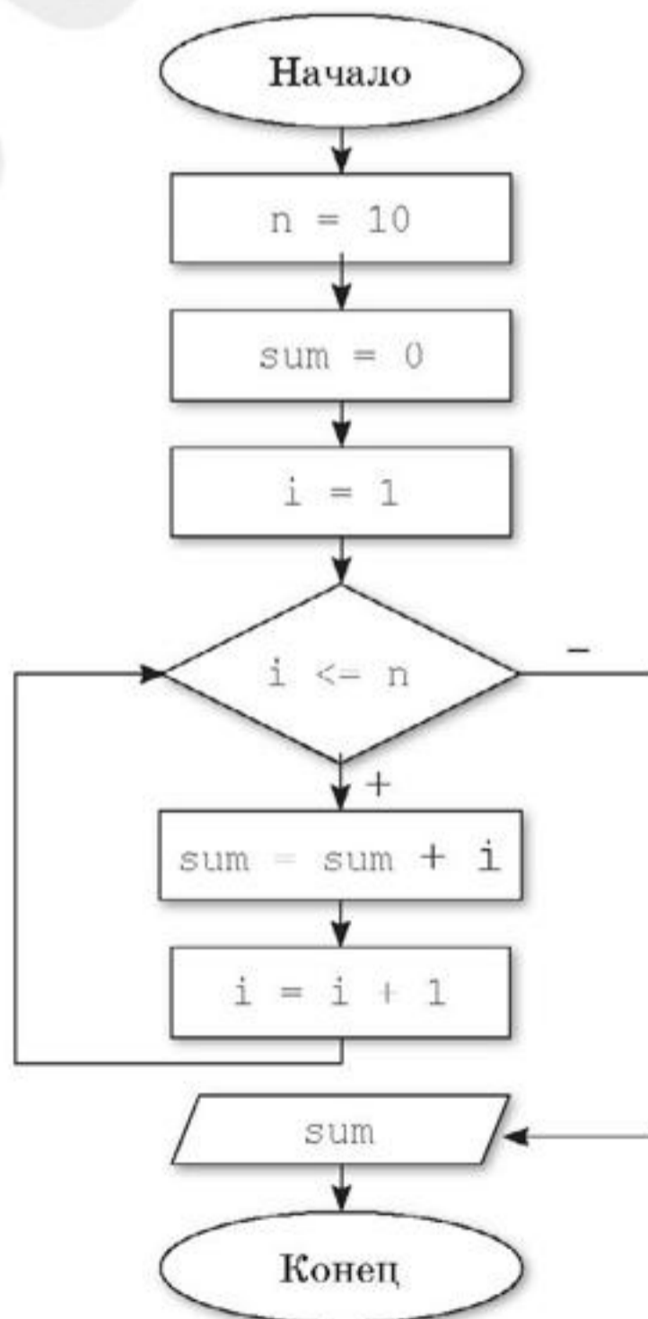
Блок-схема (Пример 2)
