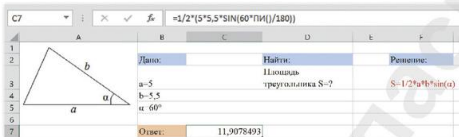
Рис. 52. Решение задачи по определению площади треугольника
