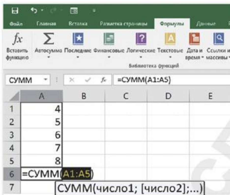
Рис. 39. Функция СУММ()
