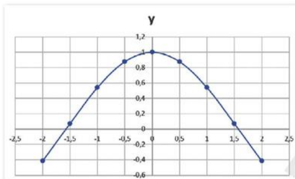
Рис. 55. График функции y = \cos x
